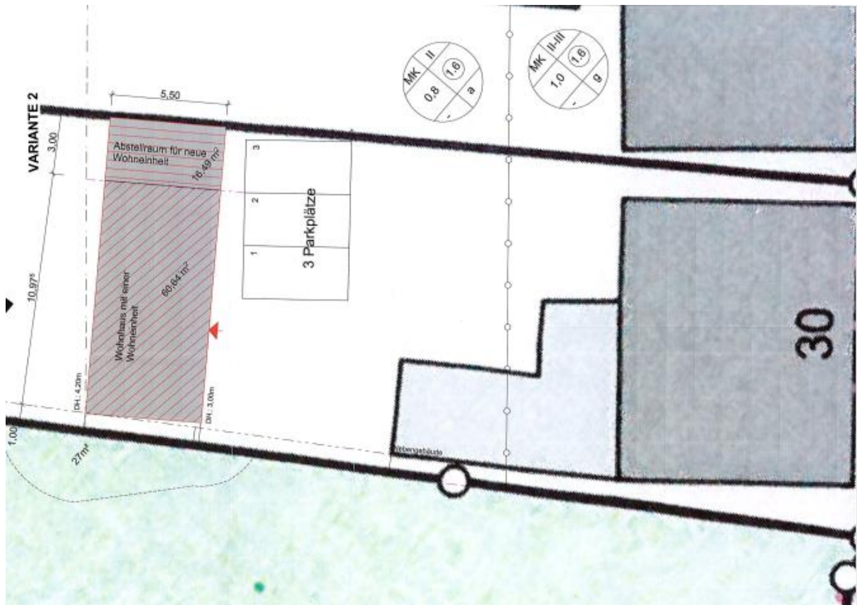
Variante 2 (unmaßstäblich)
